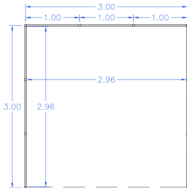
Vista planta
